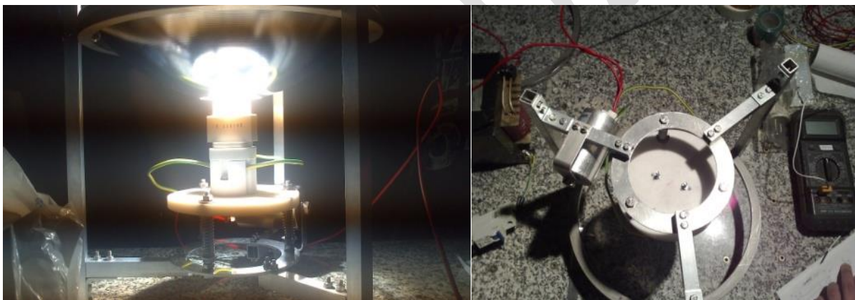
Figure 3-1 "Słonecznik" Sun simulator
